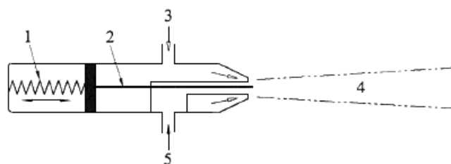
Рисунок D.1 - Форсунка
