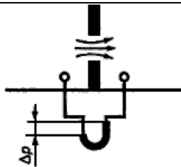
Рисунок А.7 - Принцип перепада давления
