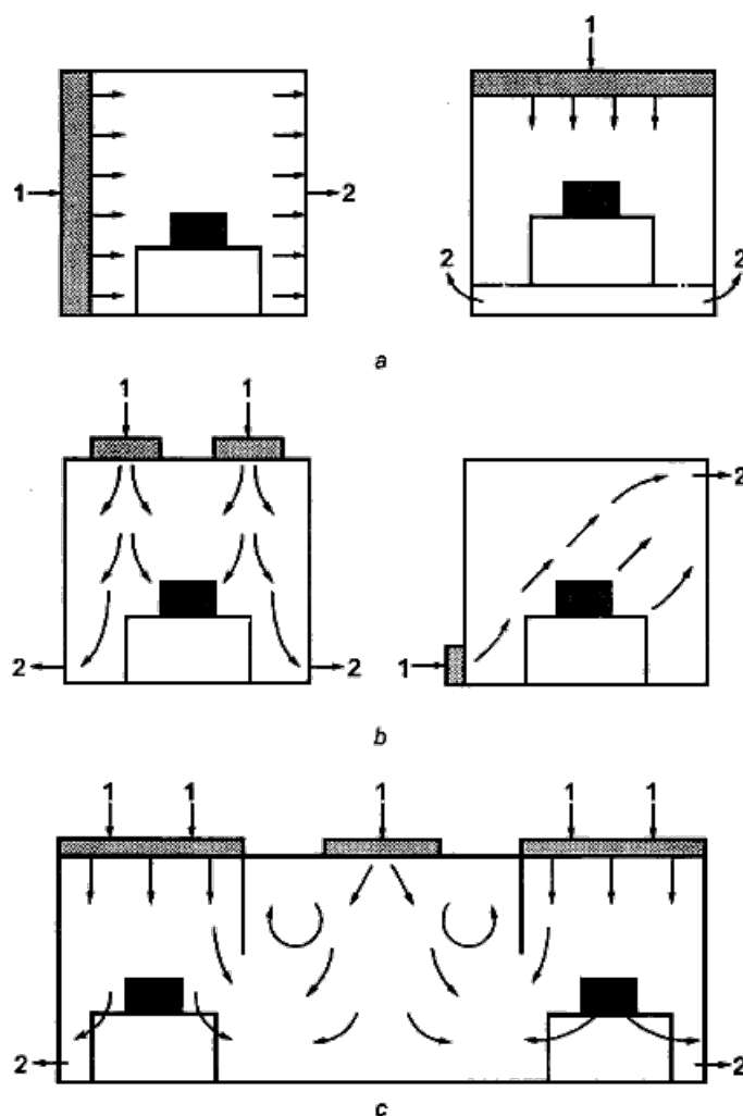
а - одинаправленный поток воздуха; б - неоднаправленный поток воздуха; с - смешанный поток воздуха; 1 - приточный воздух; 2 - вытяжной воздух
