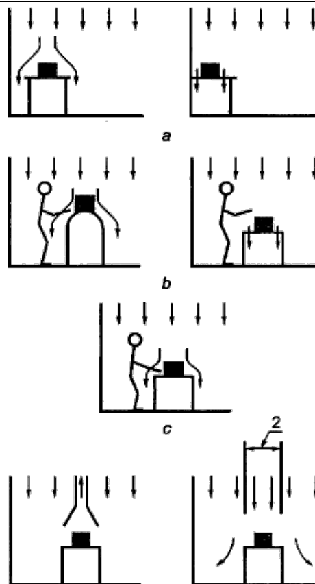
a - за счет лучшего расположения оборудования; b - за счет лучшей формы оборудования и рабочего места; c - за счет правильного поведения персонала; d - за счет специальной организации потоков воздуха; 1 - источник тепла; 2 - локальный поток с повышенной скоростью
